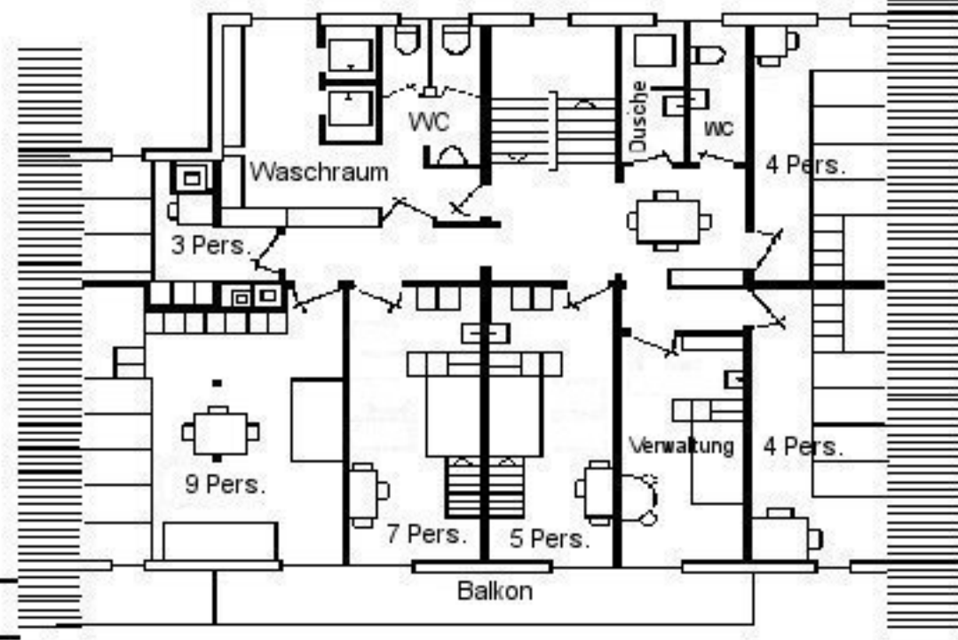
Dachgeschoss
